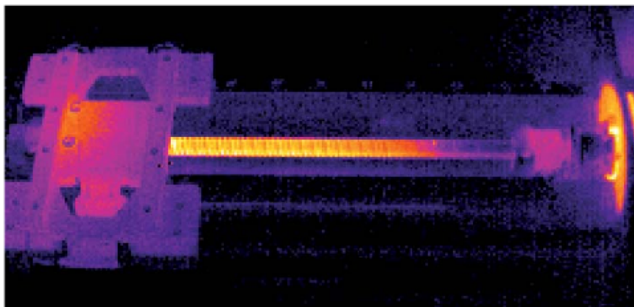
Figure 1 Echauffement d'une vis à billes lors d'une opération de fraisage ligne à une avance moyenne de 10 m/min. L'enregistrement thermographique signale des températures de 25 °C à 40 °C.
